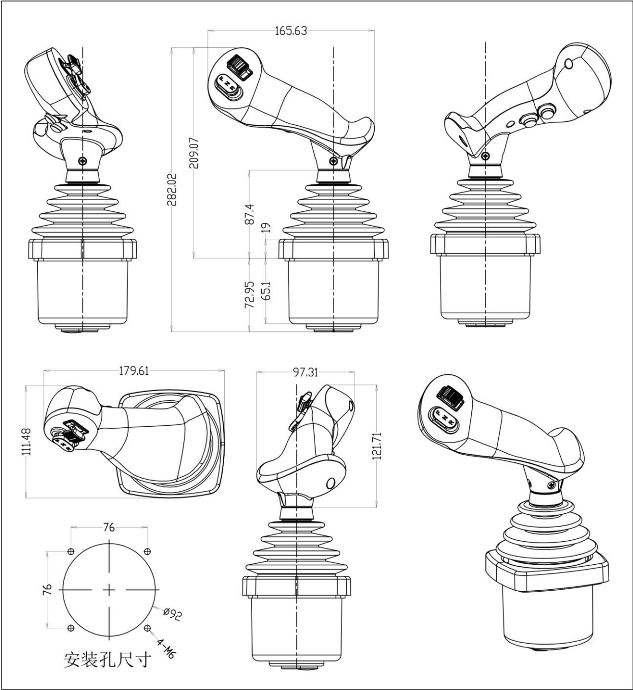
产品尺寸图:
